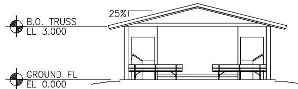
END ELEVATION
